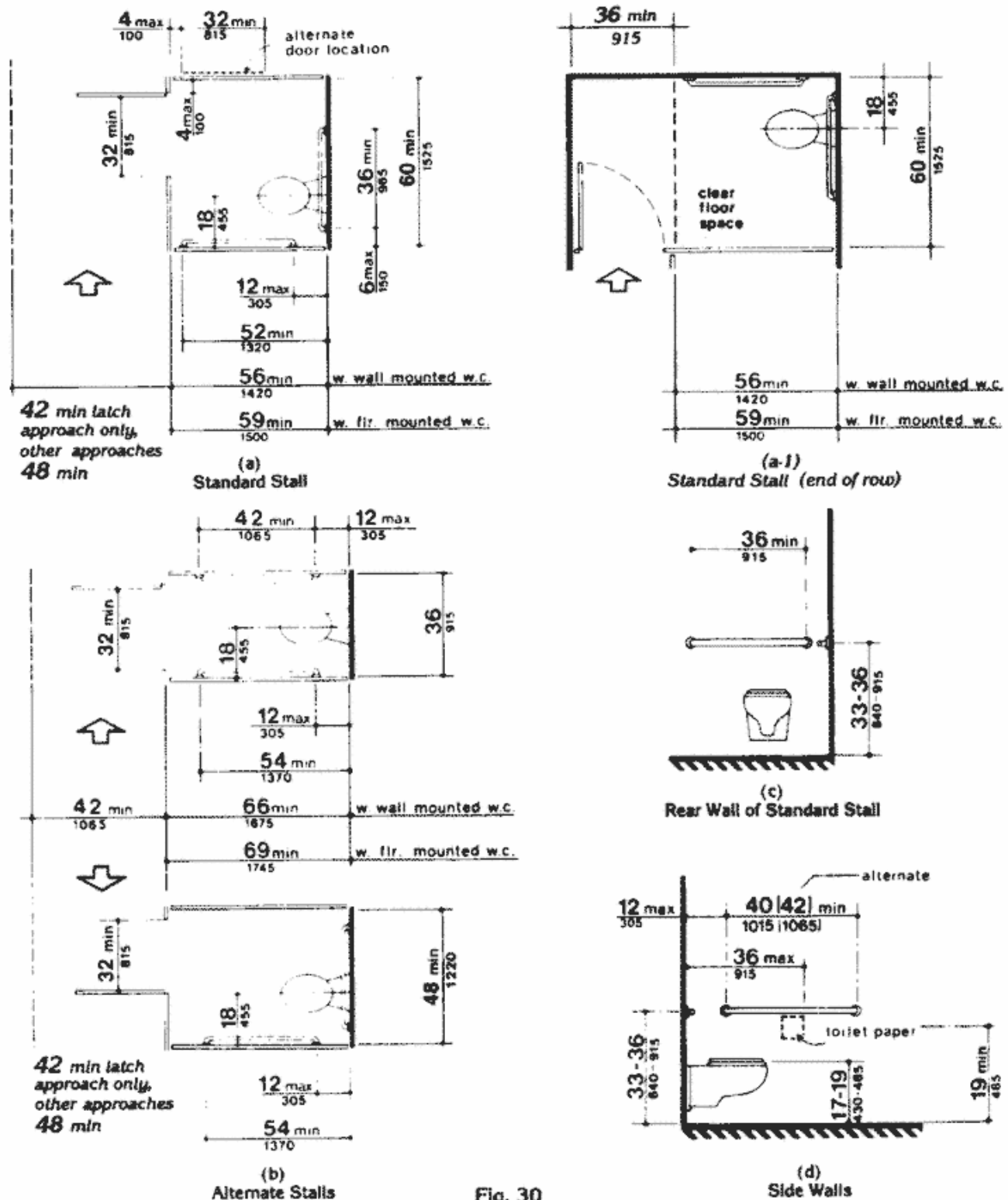
Fig. 30 Toilet Stalls
